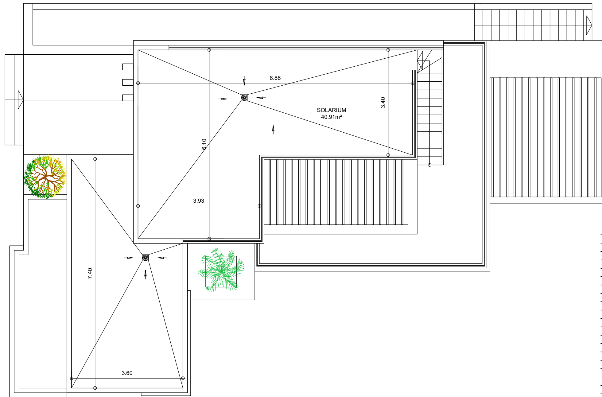
PLANTA CUBIERTA
